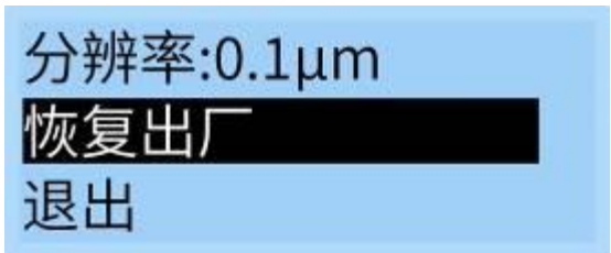
设置主界面
